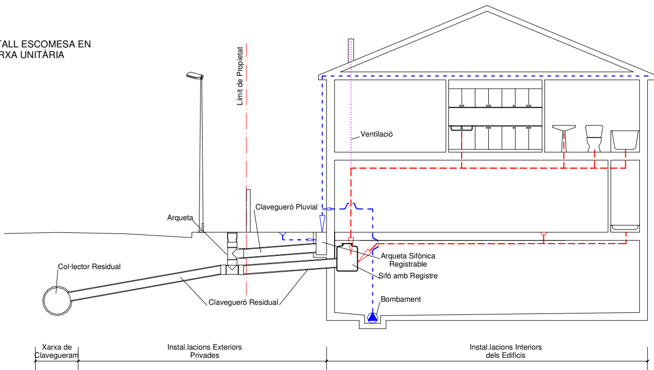
DETALL ORIENTATIU SIFÓ AMB REGISTRE
